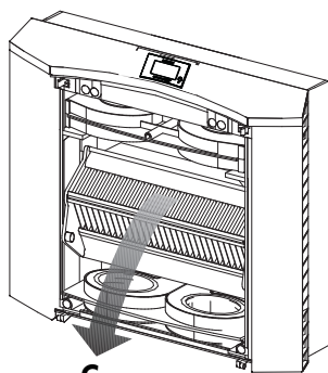
Bild 8 Wärmetauscher ausklappen
