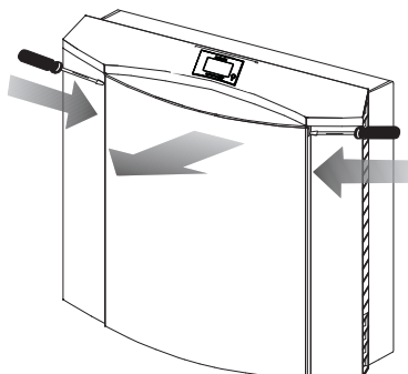
Bild 7 Frontplatte entfernen
