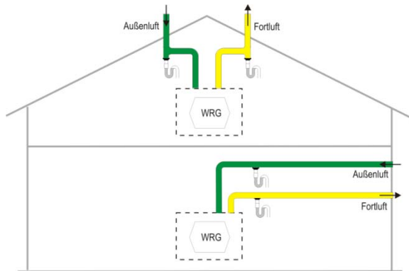
Abb. 24: Anordnung Entwässerung der Außen- und Fortluftleitung
