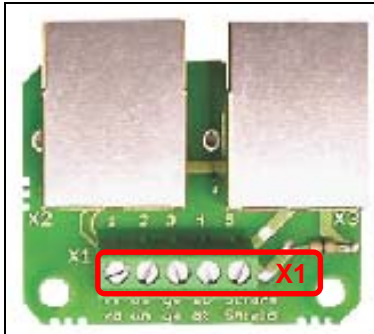
Abb. 26: Adapterplatine
