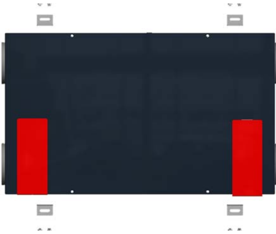
Abb. 16: Anbringen der Montagewinkel
