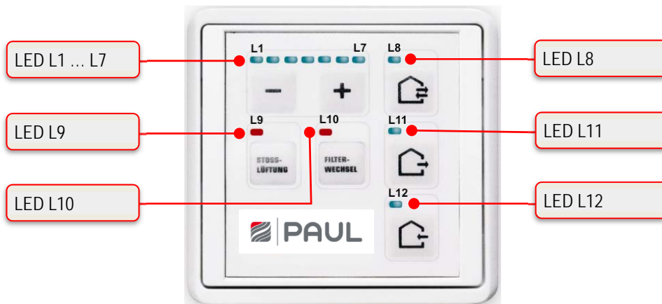
Abb. 3: LED-Signalisierungen LED-Bedienteil
