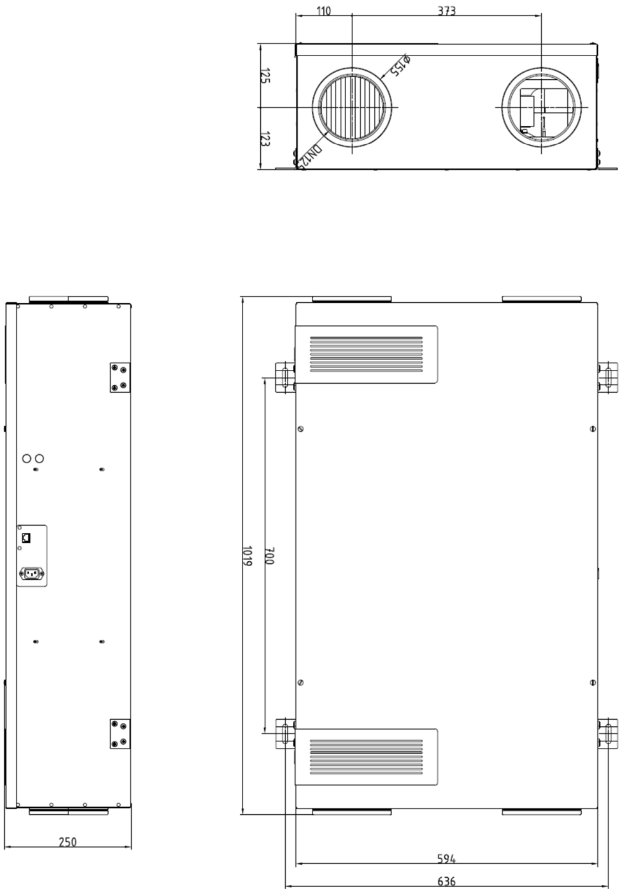
Abb. 55: Maßskizze CLIMOS
