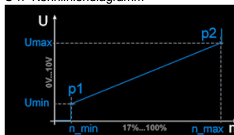
U-n- Kennliniendiagramm
