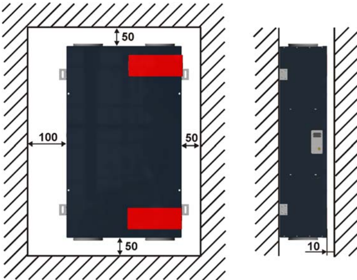
Abb. 15: Abstände in mm zu angrenzenden Flächen
