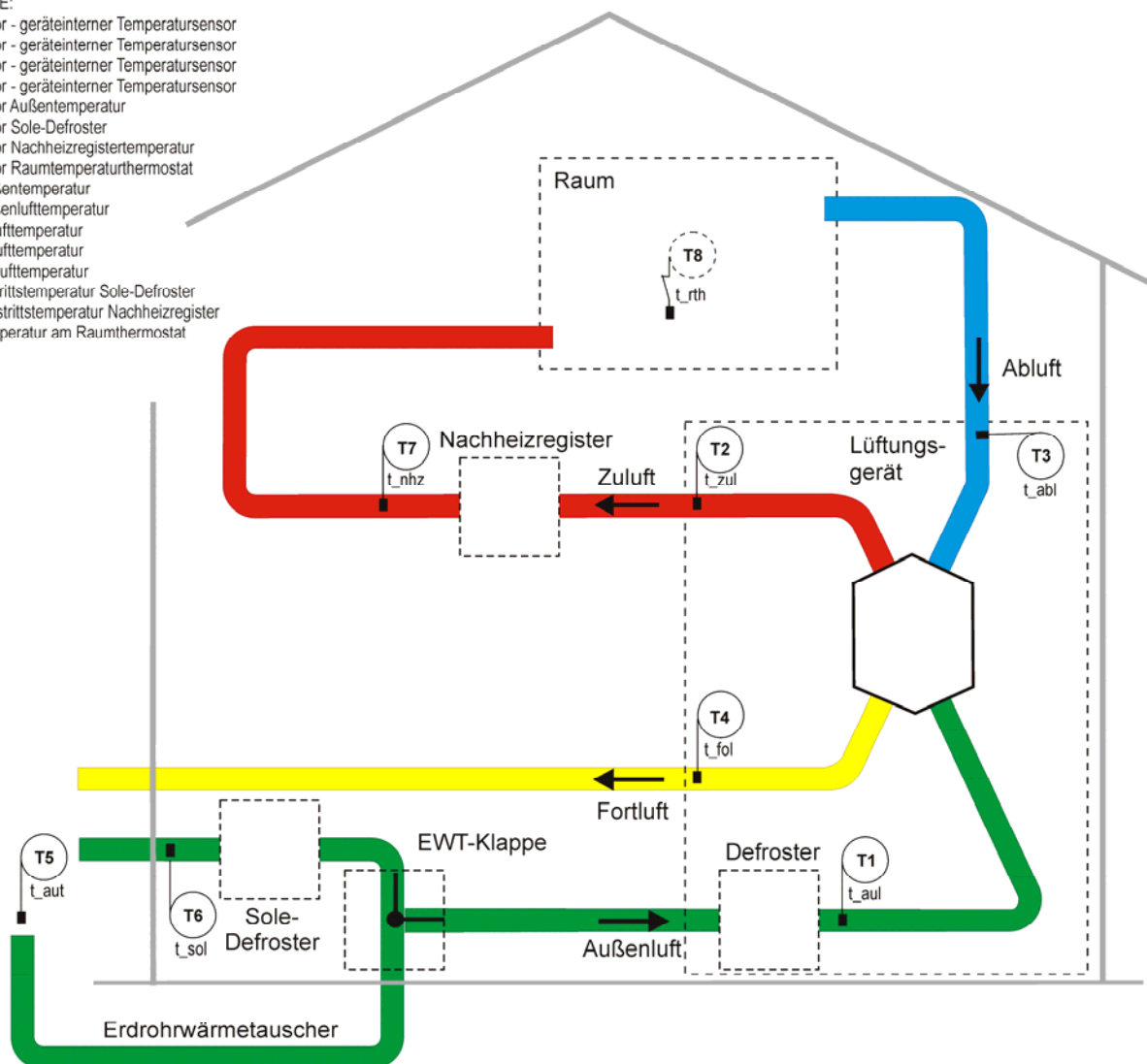
Abb. 14: Allgemeines Anlagenschema mit WRG CLIMOS F 200 Comfort - Serie
