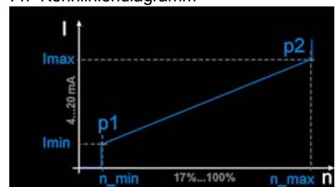
I-n- Kennliniendiagramm
