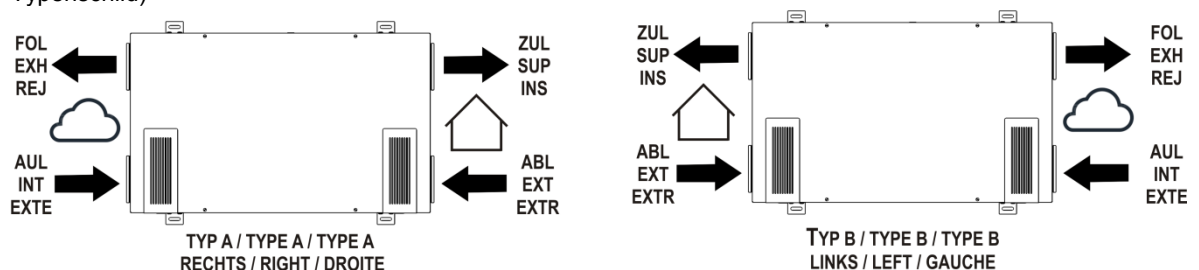
Abb. 23: Anordnung Luftanschlüsse je nach Bauform R (rechts - Typ A) / L (links - Typ B)
