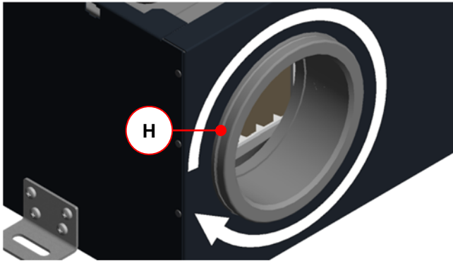
Abb. 50: Kürzen des EPP-Anchlusstutzens an der Soll-Trennstelle der umlaufenden Rille
