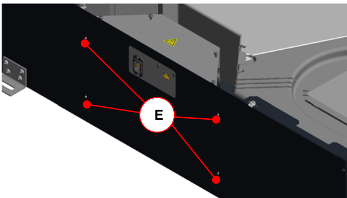
Abb. 41: Herstellen der Schlüssellochverbindung
