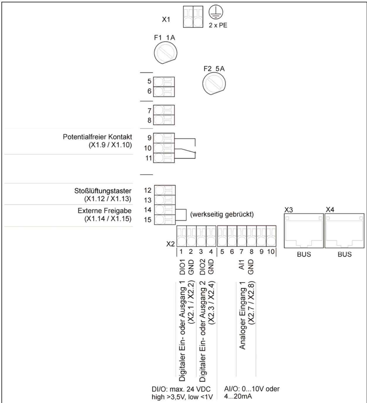
Abb. 58: Klemmenbelegung Master-Controller
