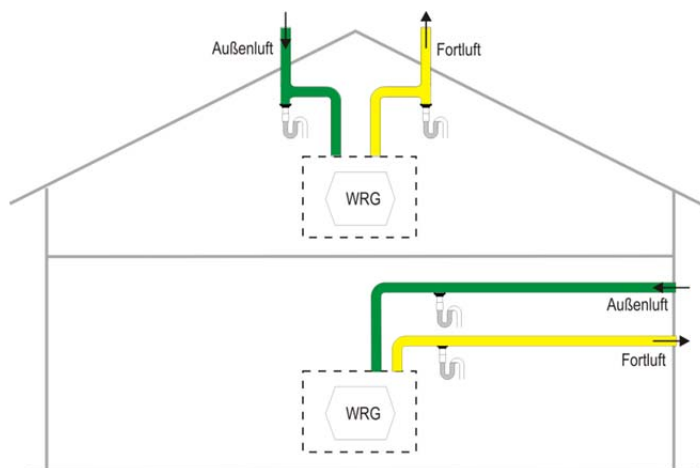
Abb. 30: Anordnung Entwässerung der Außen- und Fortluftleitung
