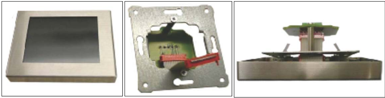
Abb. 38: Touchpad mit Edelstahlrahmen; Bandkabel der Anschlussplatine; Touchpad mit Edelstahlrahmen in UP-Tragplatte eingerastet (von links nach rechts)
