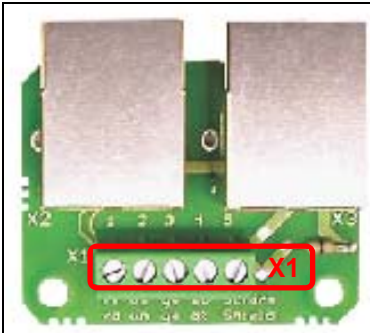
Abb. 35: Adapterplatine
