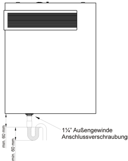
Abb. 32: Kondensatanschluss (Version LINKS, Bauart STEHEND)
