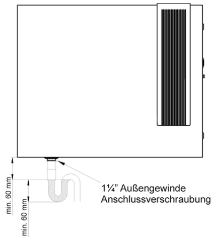
Abb. 33: Kondensatanschluss (Version RECHTS, Bauart LIEGEND)
