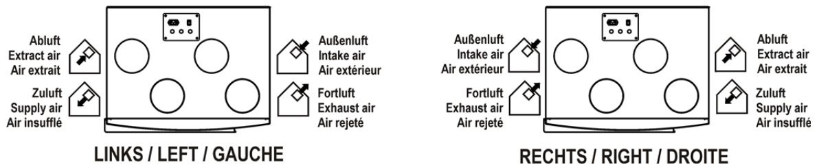
Abb. 29: Anordnung Luftanschlüsse Geräteversion LINKS und Geräteversion RECHTS
