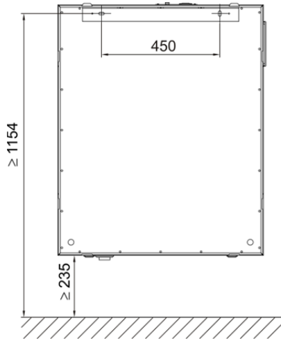
Abb. 19: Einbaulage vertikal (Version RECHTS)
