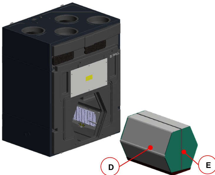
Abb. 45: Entnehmen des Wärmetauschers
