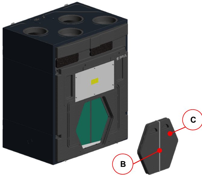
Abb. 44: Entnehmen der EPP-Wärmetauscherabdeckung
