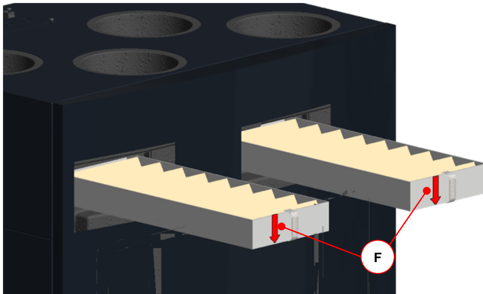
Abb. 15: Einsetzen der neuen Filter
