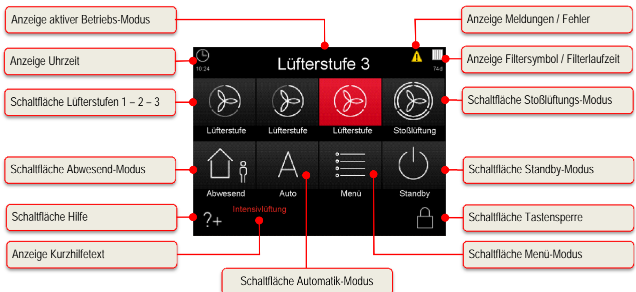
Abb. 7: Schalt- und Informationsflächen des Touchpad
