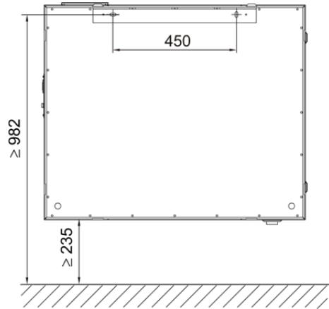
Abb. 20: Einbaulage horizontal (Version RECHTS, Bauart LIEGEND – RECHTS)
