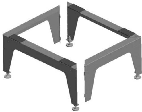
Abb. 26: Je zwei miteinander fixierte Fußteile
