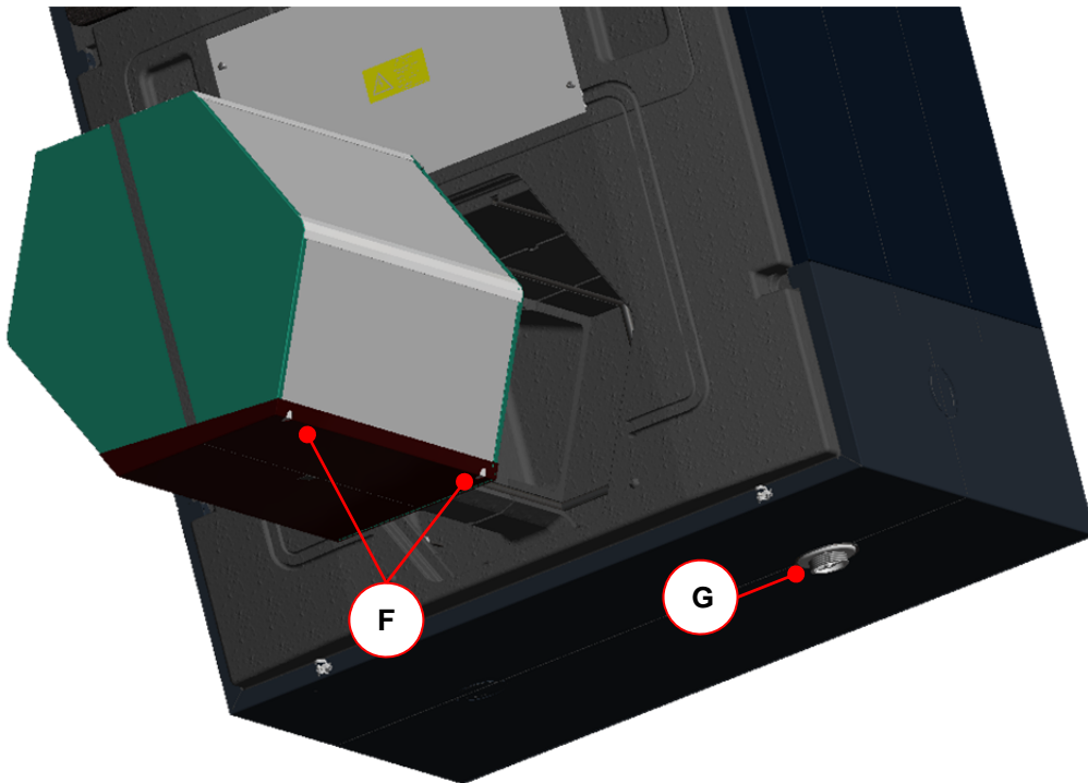
Abb. 46: Einschieben des Wärmetauschers bezüglich der Ausrichtung der Aussparungen an der Kondensatwanne
