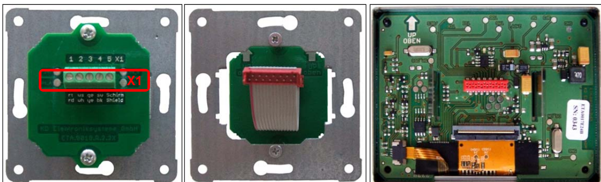
Abb. 37: Anschlussplatine mit Klemme X1 auf UP-Tragplatte; Bandkabel der Anschlussplatine; Platine TFT-Touchpanel (von links nach rechts)
