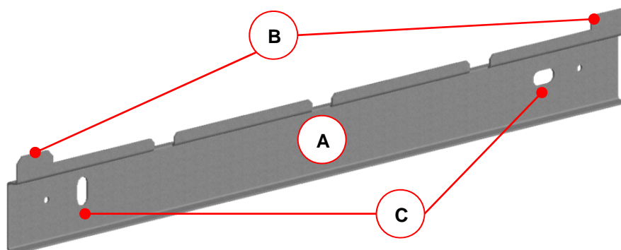
Abb. 18: Befestigungsblech für Wandmontage
