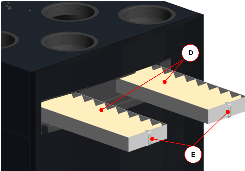
Abb. 14: Entnahme der Filter
