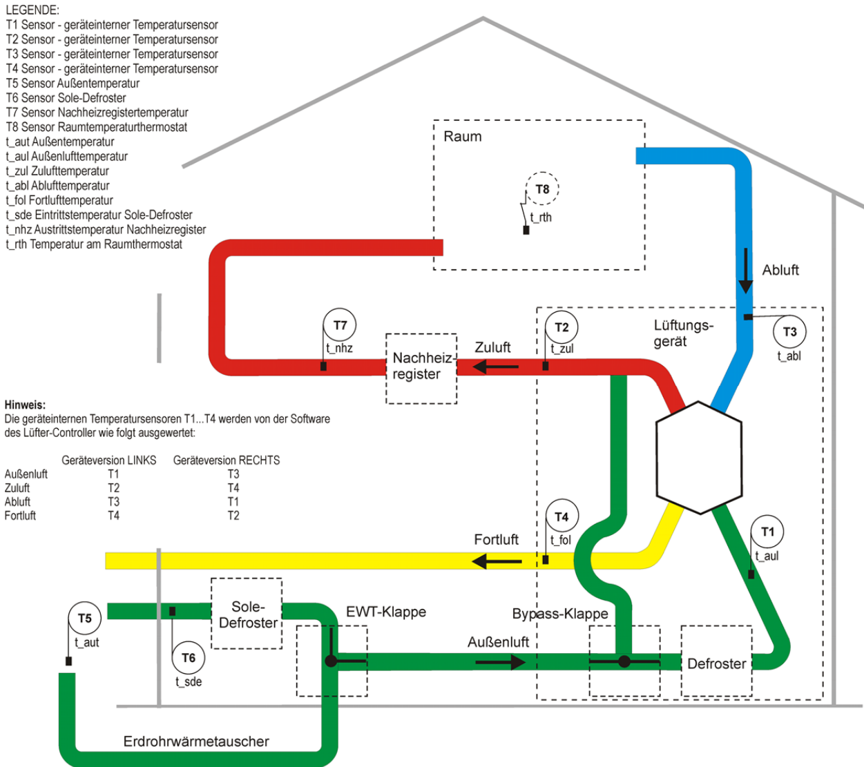
Abb. 17: Allgemeines Anlagenschema mit WRG NOVUS und integrierten Defroster, Version LINKS
