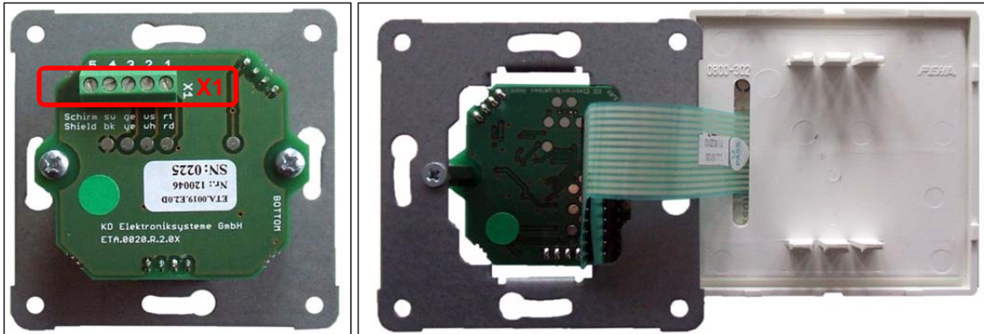
Abb. 39: Anschlussplatine mit Klemme X1 auf UP-Tragplatte; Bandkabel der Anschlussplatine; Rückseite LED-Bedienfolie (von links nach rechts)
