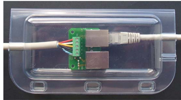
Abb. 36: Gehäuse für Adapterplatine
