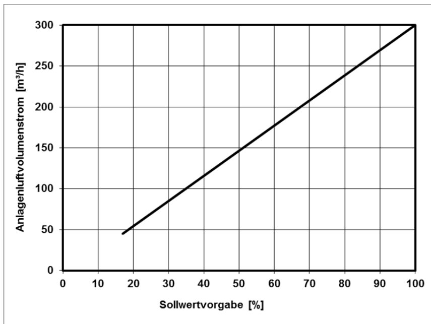
Abb. 40: Diagramm 1, Einstellwerte Nennluftvolumenstrom NOVUS (F) 300 mit Lüfterstufe 2 (LS2)
