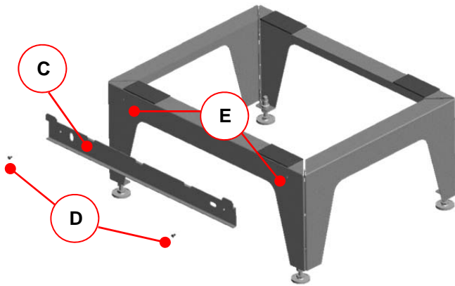
Abb. 27: Montage des Befestigungsbleches an das Fußteil
