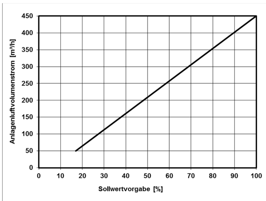
Abb. 41: Diagramm 2, Einstellwerte Nennluftvolumenstrom NOVUS (F) 450 mit Lüfterstufe 2 (LS2)
